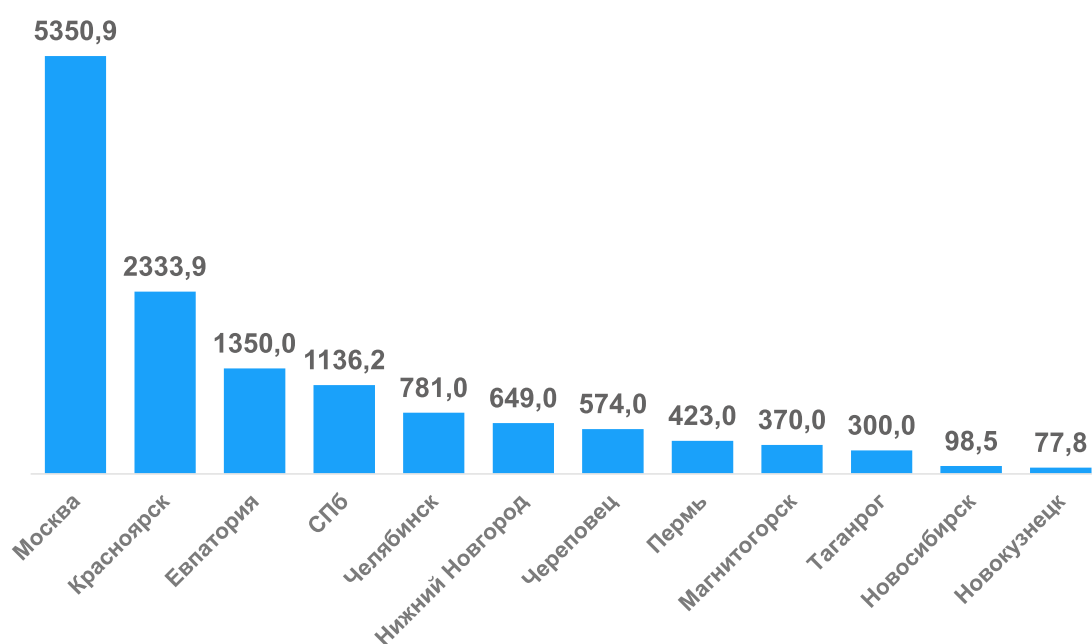
Рисунок 9. Объемы закупок трамвайных вагонов в разрезе городов в 2021 г. в стоимостном выражении, млн руб.
