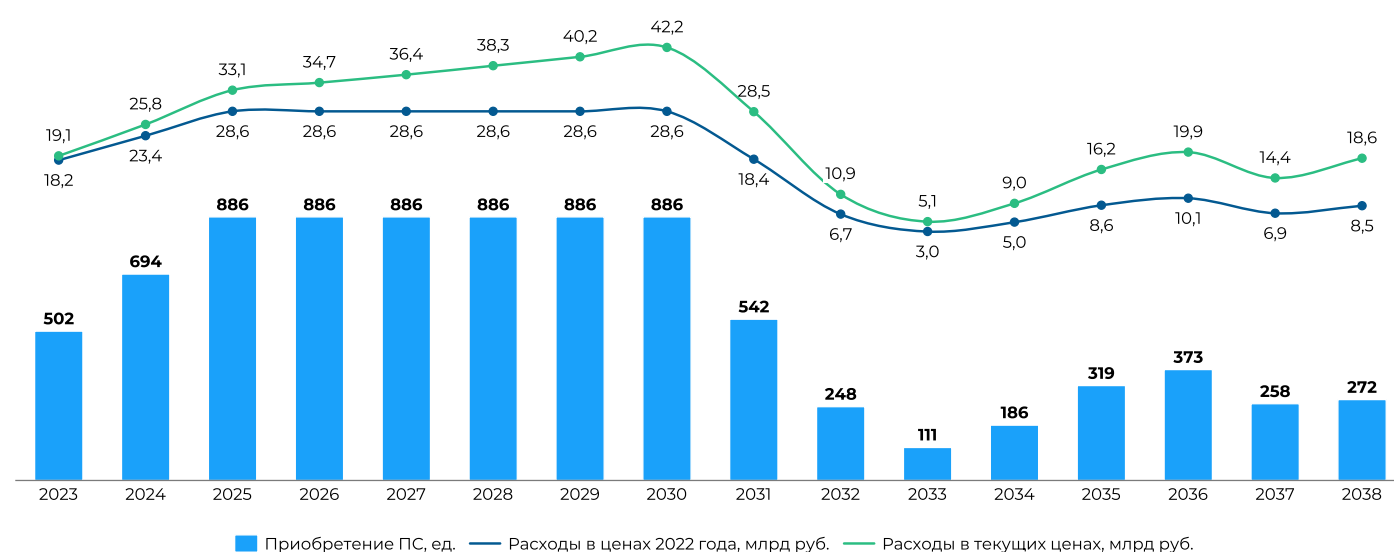
Рисунок 23. График закупки троллейбусов на период до 2038 г. (план)
