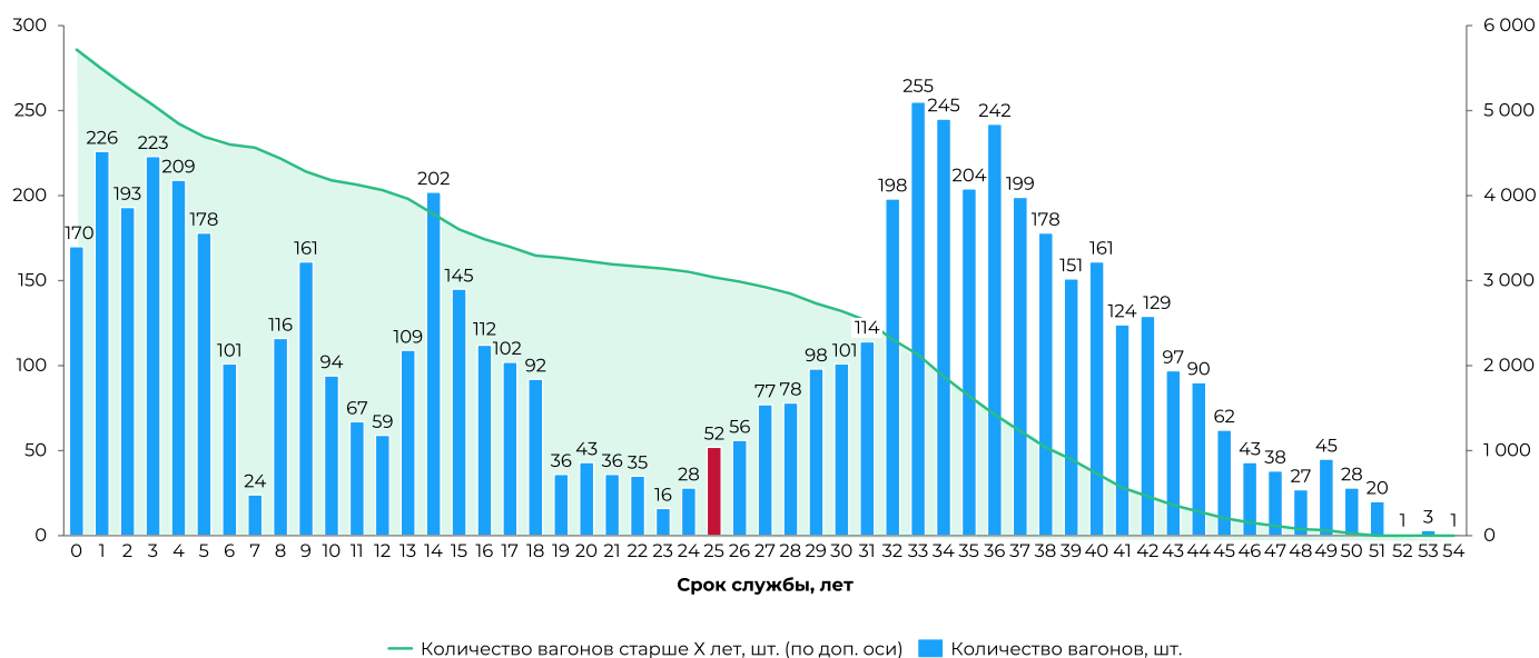
Рисунок 22. Распределение парка трамвайных вагонов по сроку эксплуатации в 2022 г.
