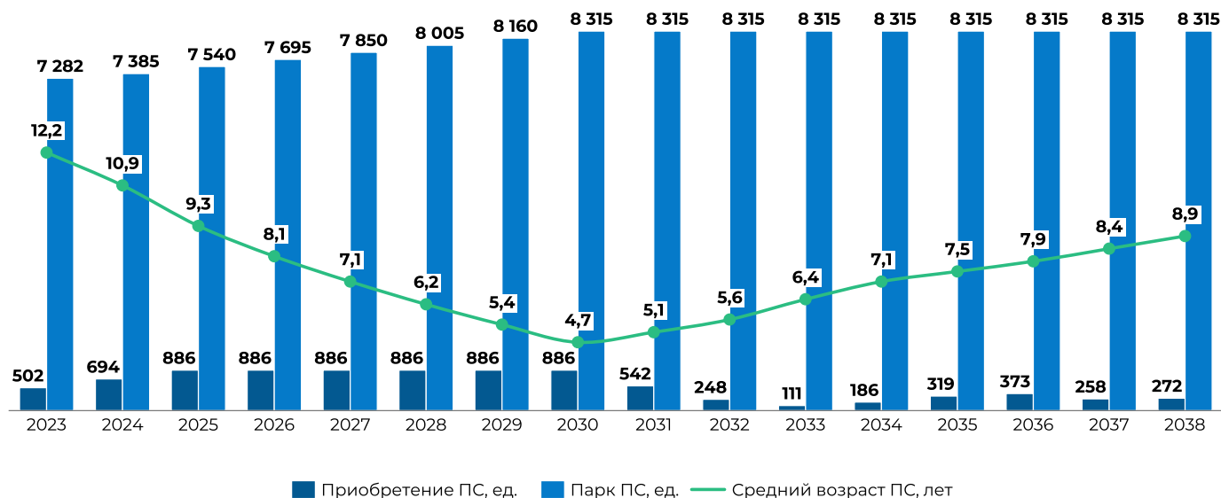
Рисунок 24. Динамика парка и среднего возраста троллейбусов на период до 2038 г.
