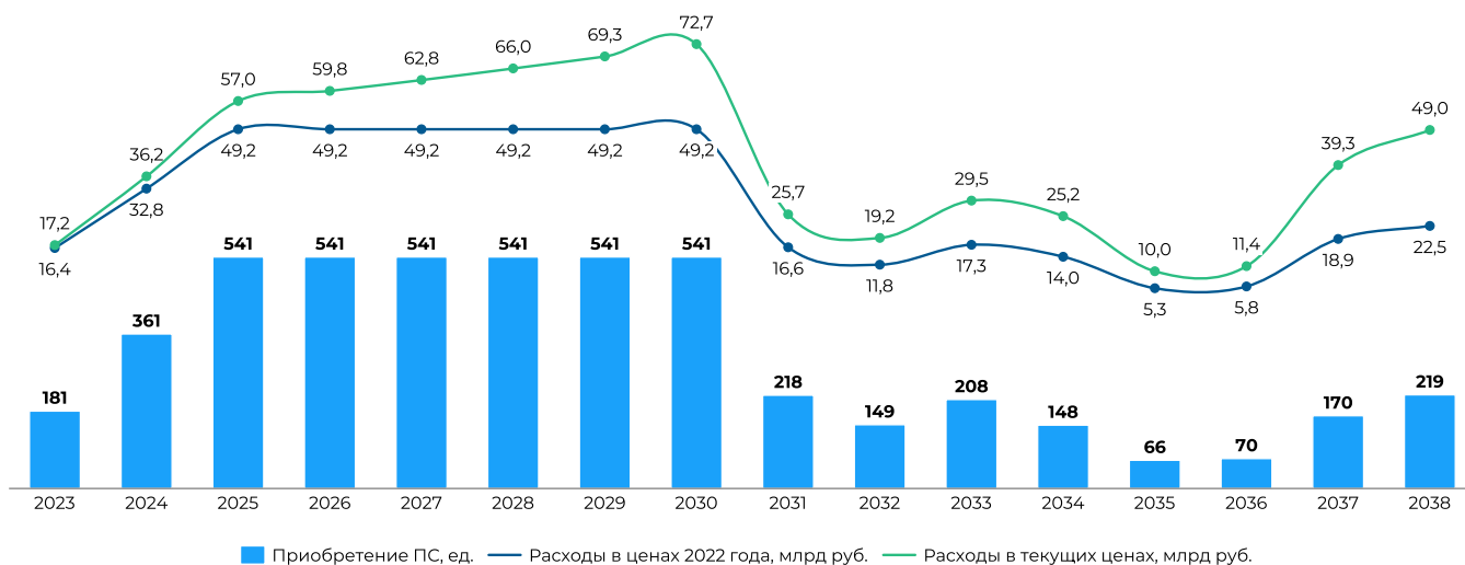
Рисунок 25. График закупки трамвайных вагонов на период до 2038 г. (план)
